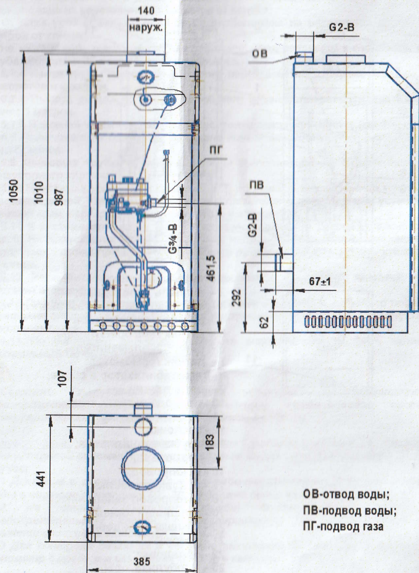
Рис.2 Габаритные и присоединительные размеры аппарата АОГВ 29-1
