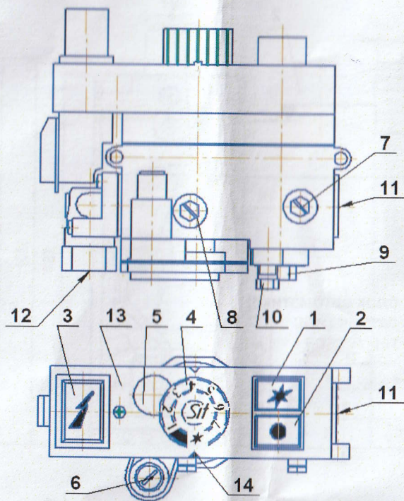
Рис.4 Элементы управления и регулировки газового клапана
