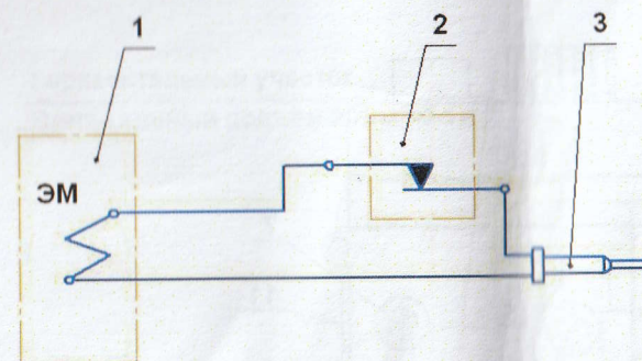
Рис.3 Схема электрическая
