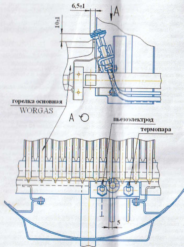
Рис.7 Схема расположения горелки запальной относительно основной (12-тигсекционной).
