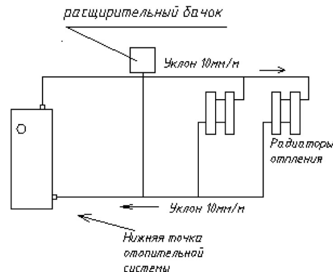
Рис.2 Схема монтажа системы отопления.
