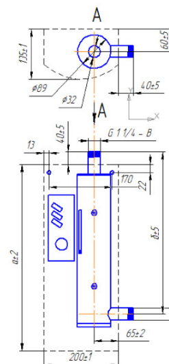
рис.1 Электроводонагреватель.
